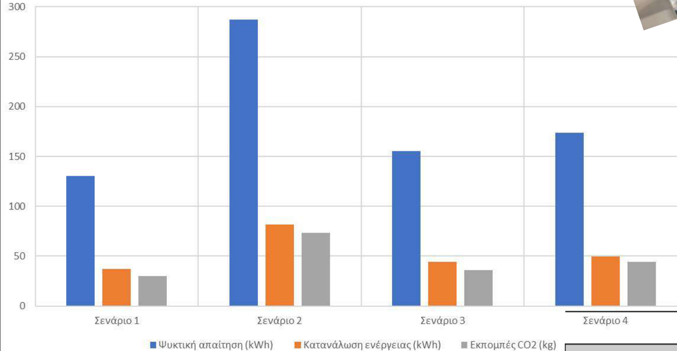
Ενεργειακή και περιβαλλοντική απόδοση των εξεταζομένων σεναρίων
