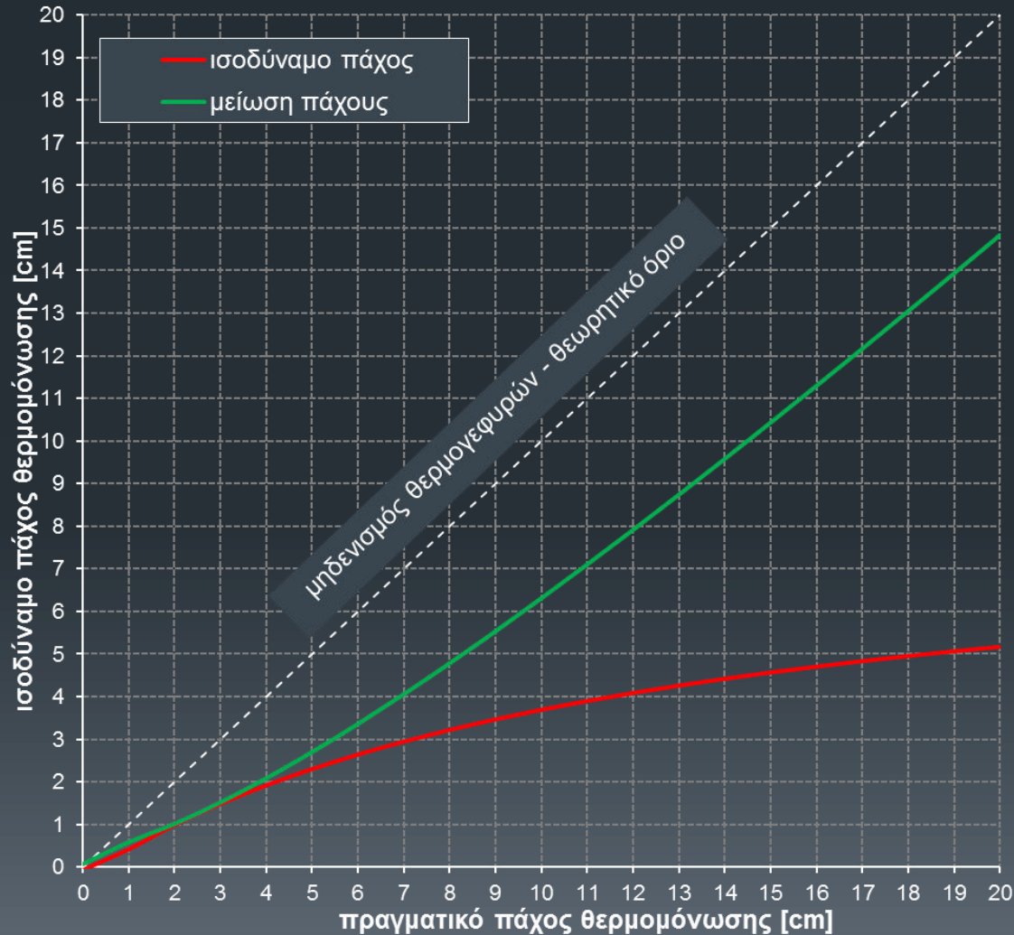
“ενεργό” πάχος θερμομόνωσης χωρίς πρόνοια μείωσης θερμογεφυρών
