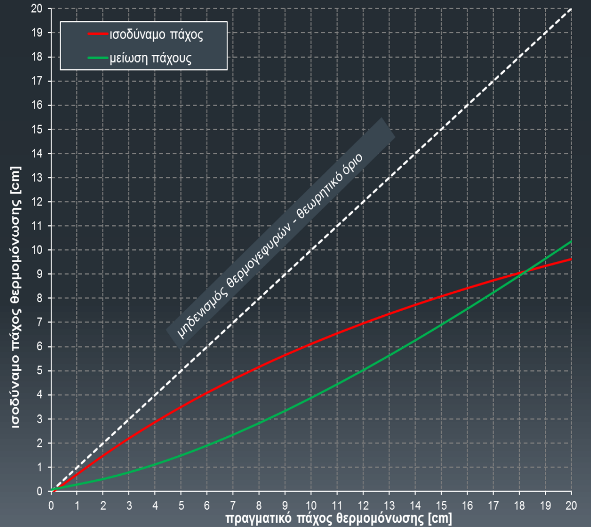
“ενεργό” πάχος θερμομόνωσης με πρόνοια μείωσης θερμογεφυρών
