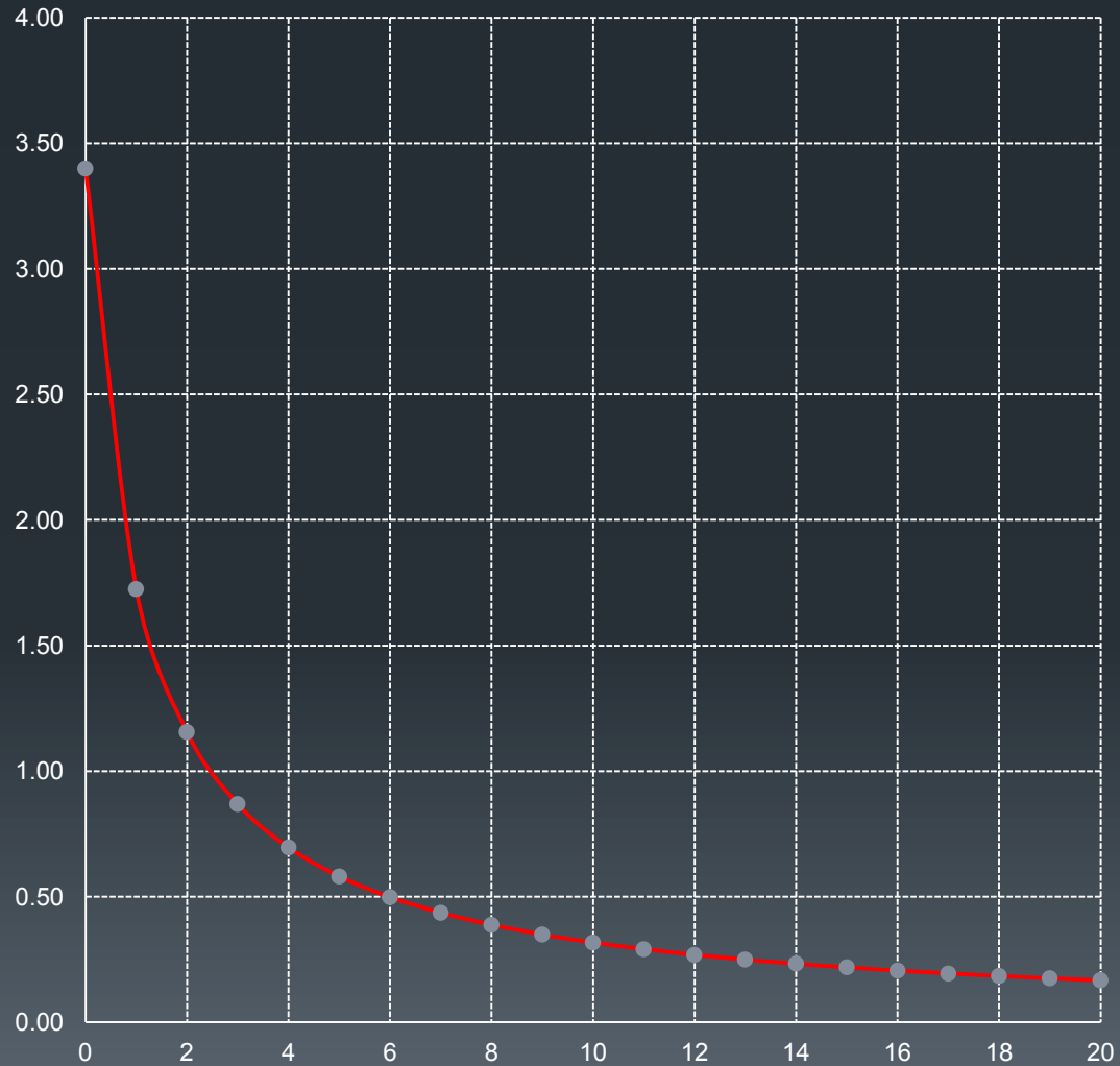
απώλειες vs πάχος μόνωσης
